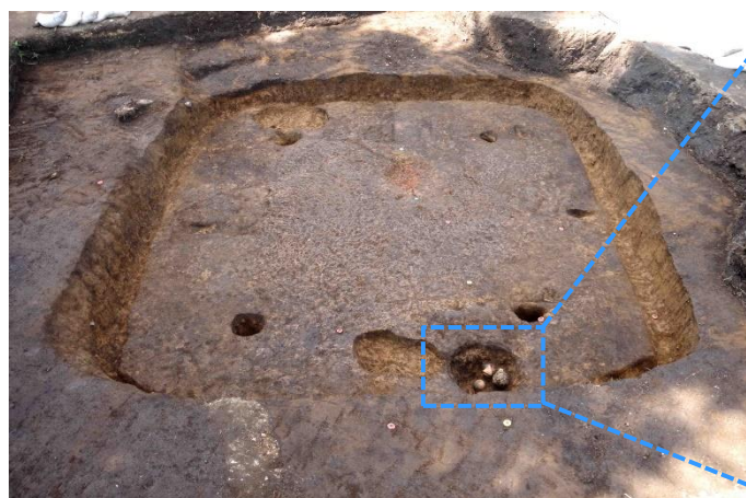
弥生時代後期～古墳時代初頭の竪穴住居跡 一辺が約5mを測る、隅が丸い方形。
