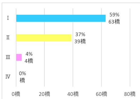
図 3-1. 健全性の集計結果 (令和 2 年点検時)
