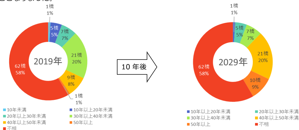
図 1-1. 供用年数別の橋梁数の推移
