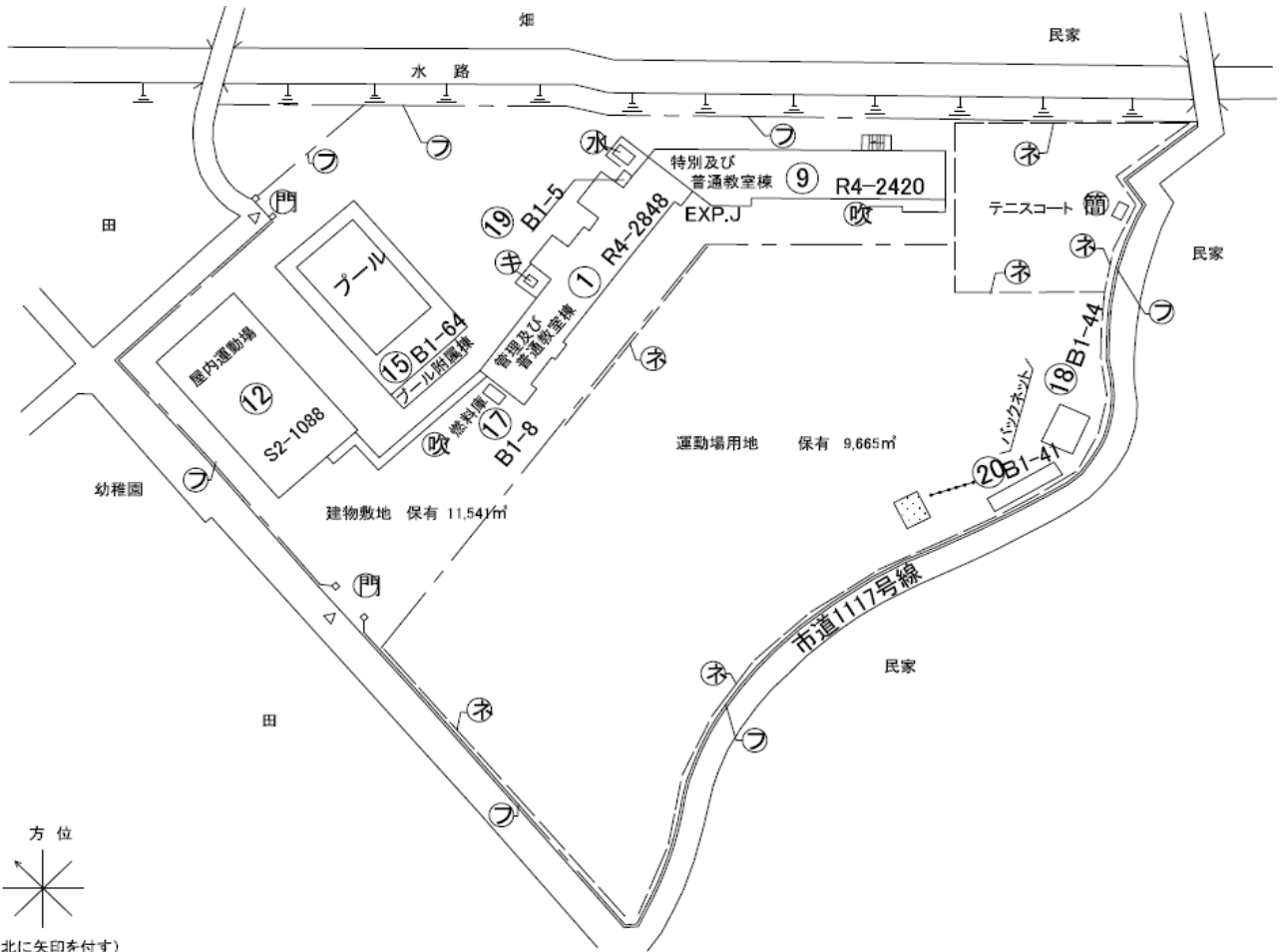
敷地・建物全体図
